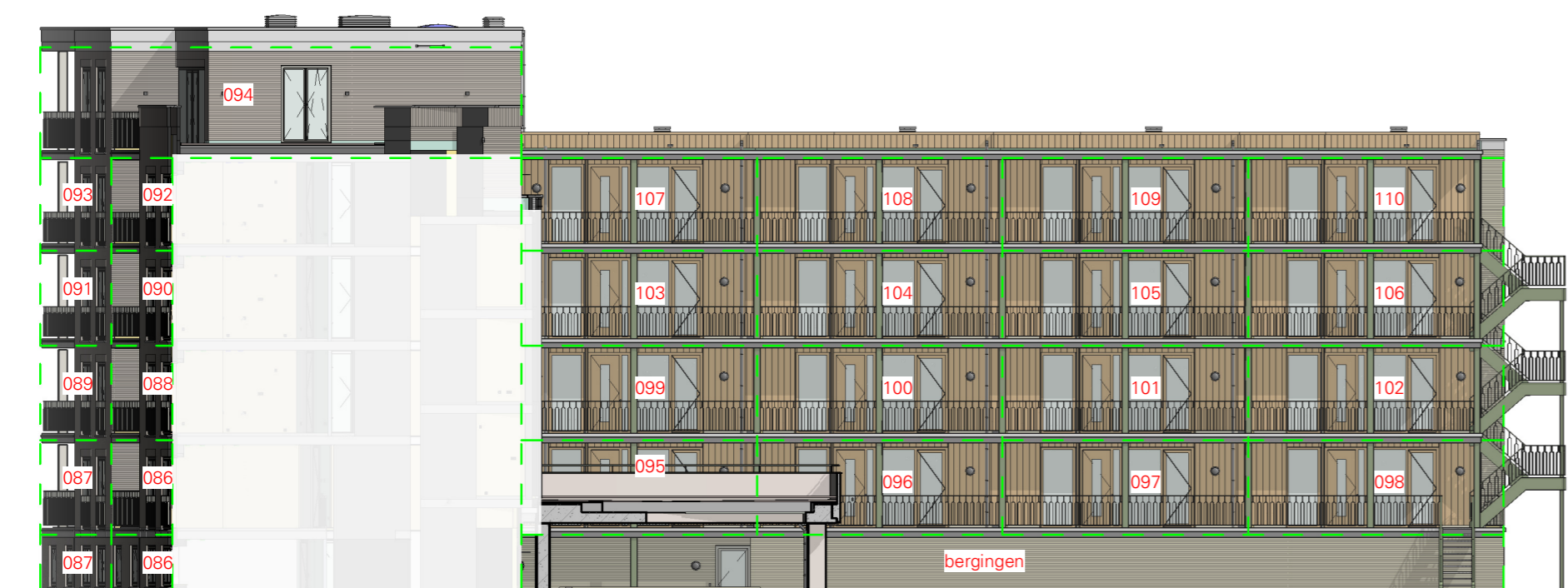
03 Zuidgevel blok 3
